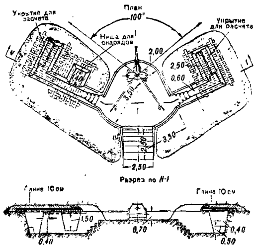
Черт. N. Окоп для 76-мм пушки с сектором обстрела 100°
