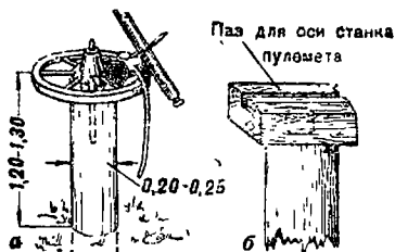
Черт. 5. Приспособление для стрельбы по воздушным целям из станкового пулемета (устанавливается на дне ячейки или за маской):
