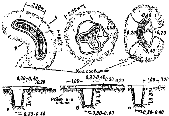
Черт. 6. Типы окопов на одно противотанковое ружье:
