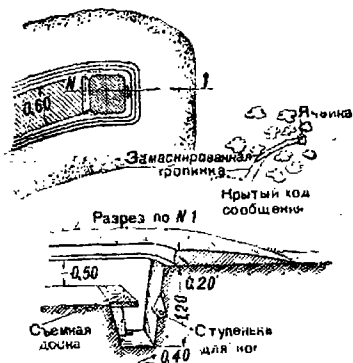
Черт. 2. Ячейка для снайпера.
