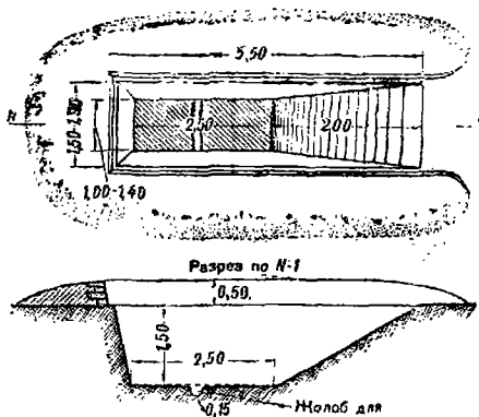
Черт. 12. Ячейка для укрытия лошади
