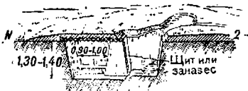
Черт. 3. Универсальная ячейка для противотанкового ружья, станкового и ручного пулемета (для станкового пулемета длина площадки — 1,4 м)
