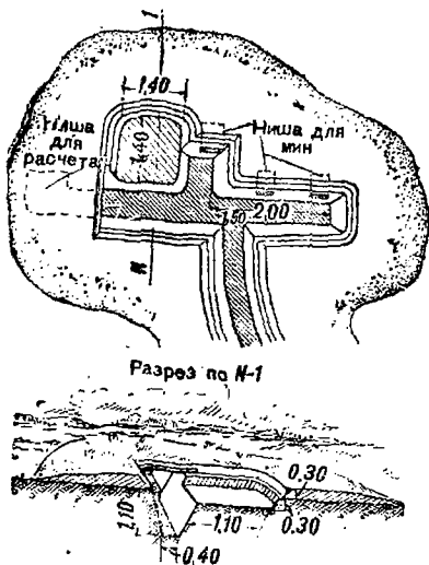
Черт. 7. Окоп для 50-мм миномета
